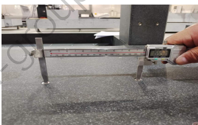
Vernier caliper
